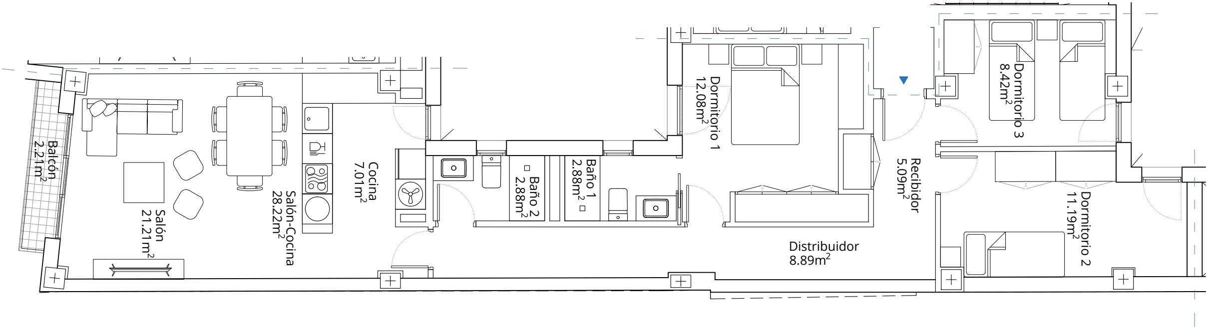
PLANTA TERCERA VIVIENDA "A"
