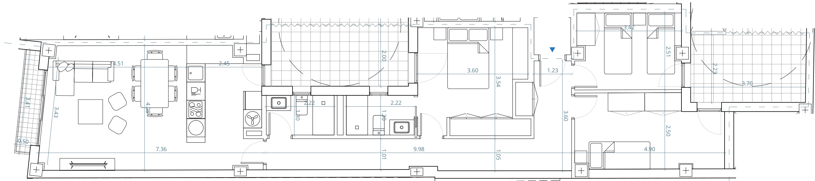
PLANTA PRIMERA VIVIENDA "A"
