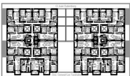
PLANTA 2 a 1.374.72 m 2 - 22 VIVIENDAS TOTAL PROYECTO 94 VIVIENDAS
