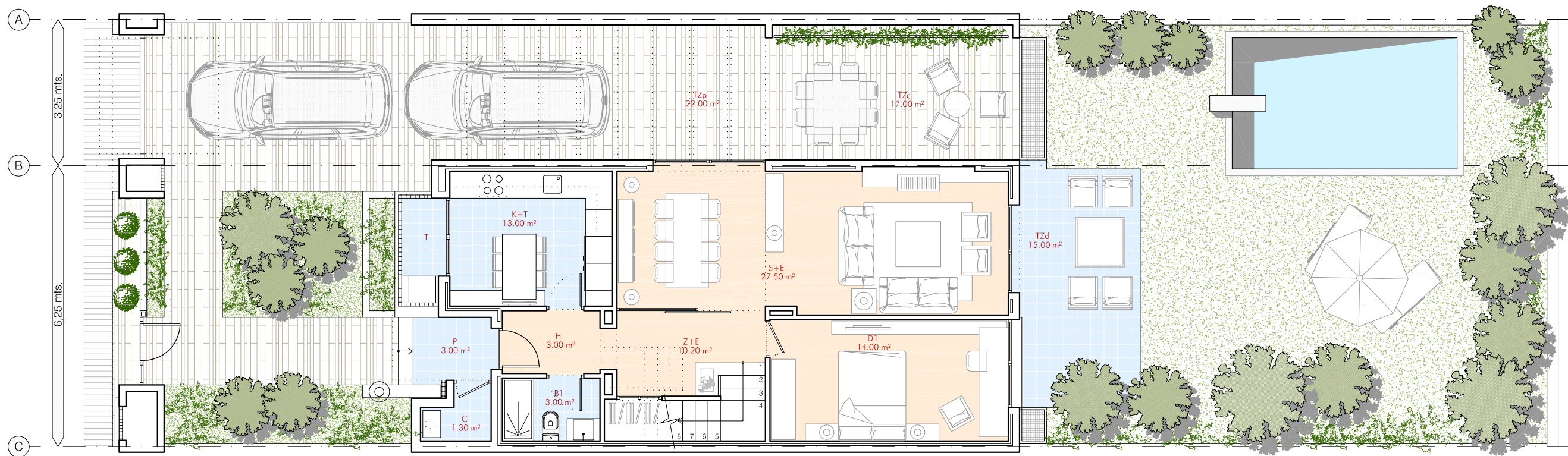
PLANTA BAJA 1/100
