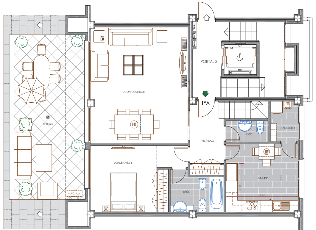
Planta INFERIOR de la Vivienda Dúplex
