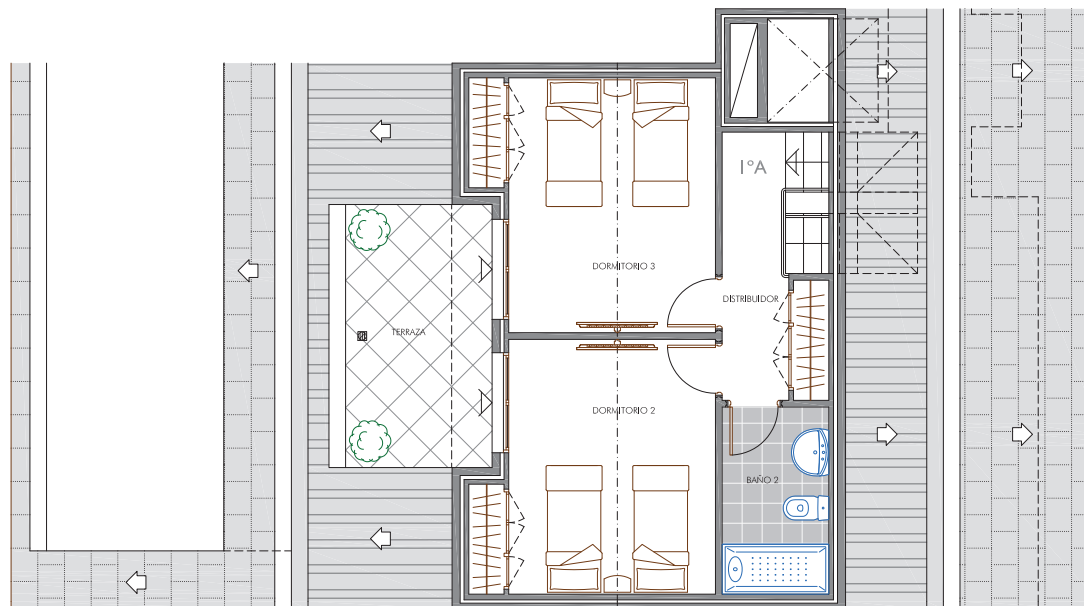
Planta SUPERIOR de la Vivienda Dúplex
