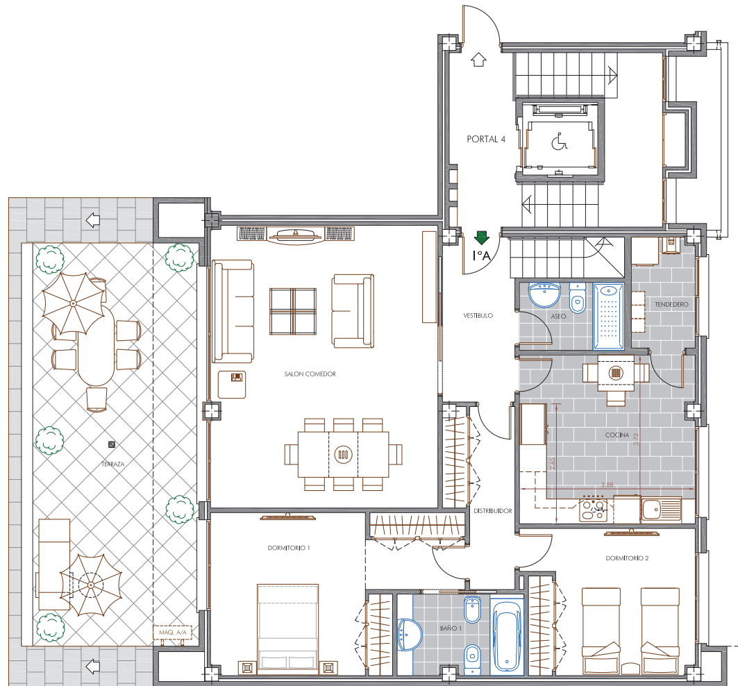
Planta INFERIOR de la Vivienda Dúplex
