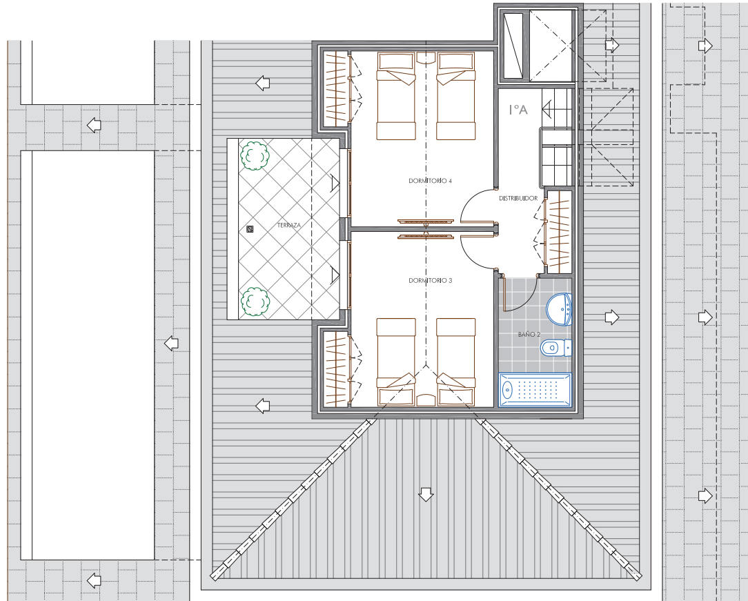
Planta SUPERIOR de la Vivienda Dúplex
