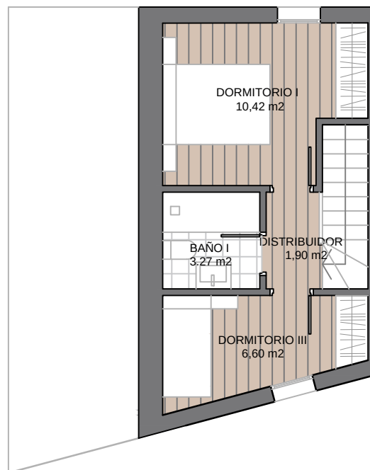
PLANTA SUPERIOR
