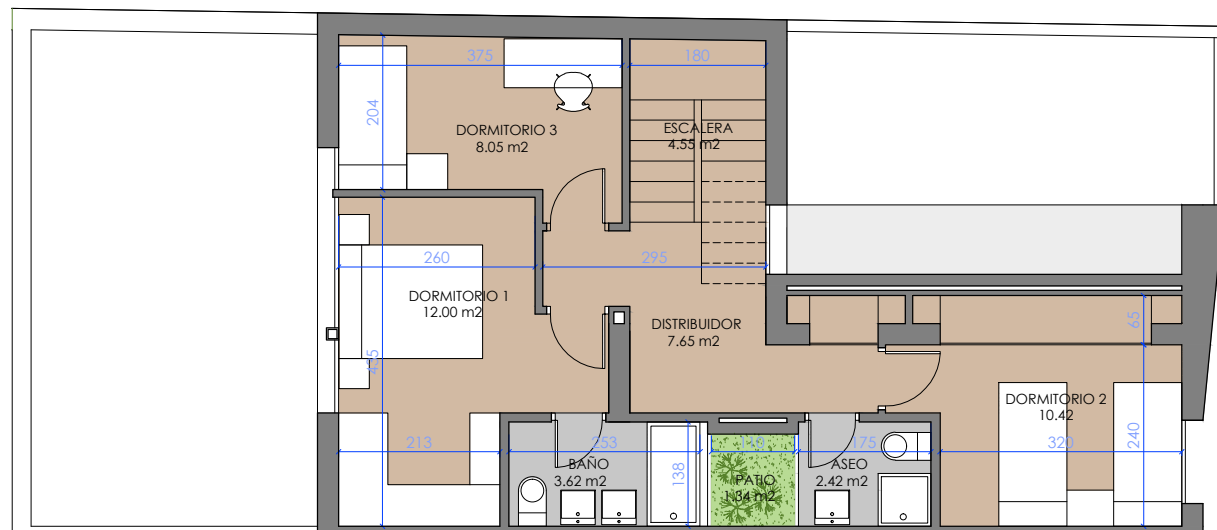
PLANTA ALTA
