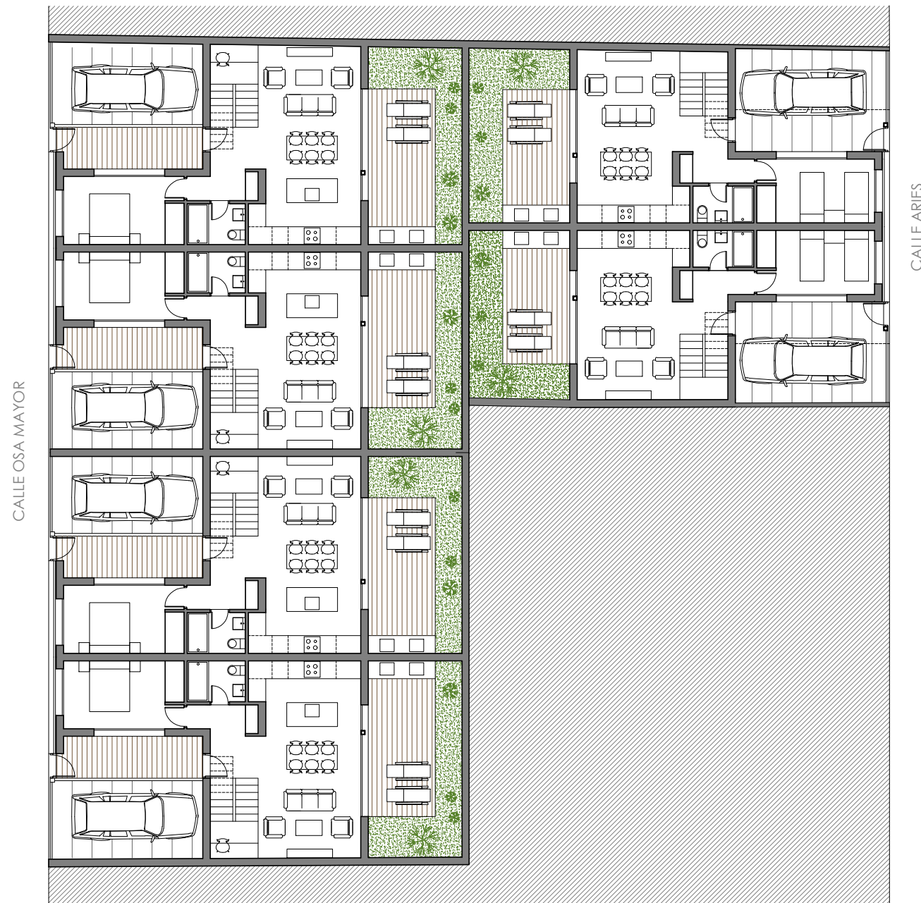
PLANTA BAJA
