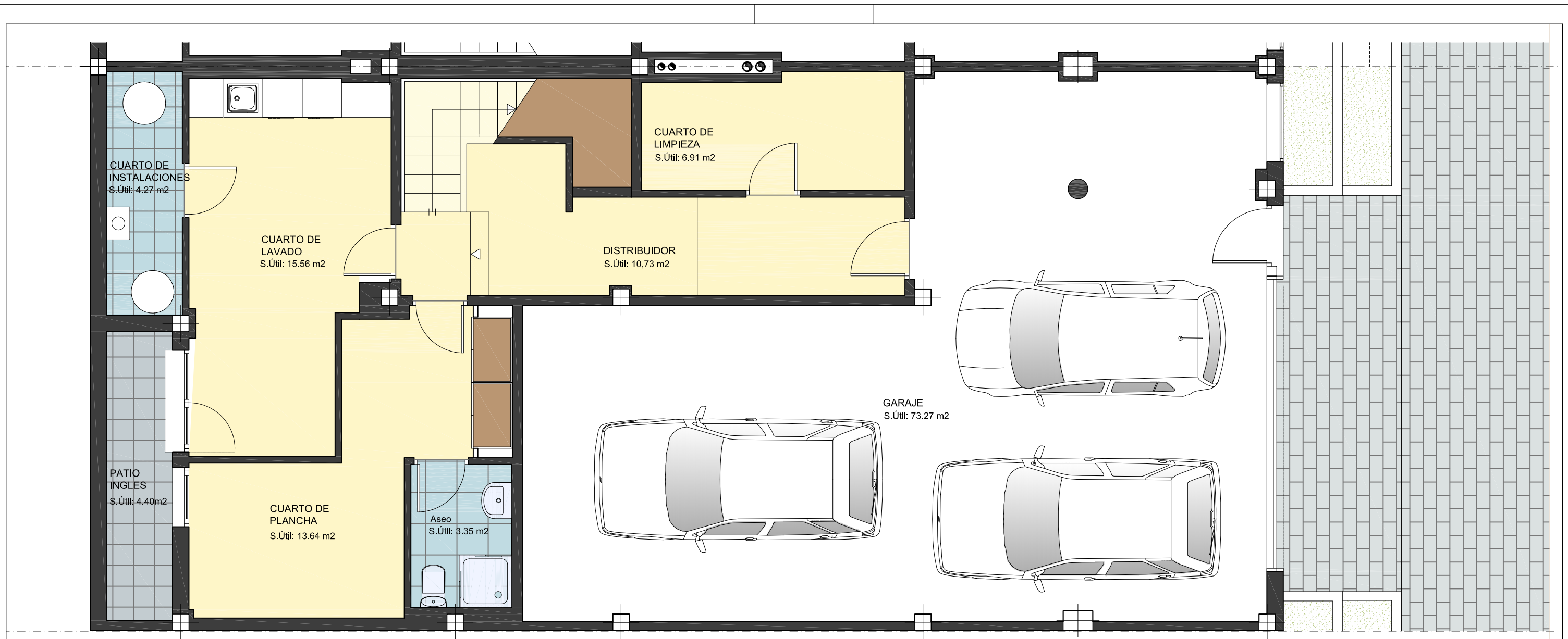
PLANTA SOTANO
