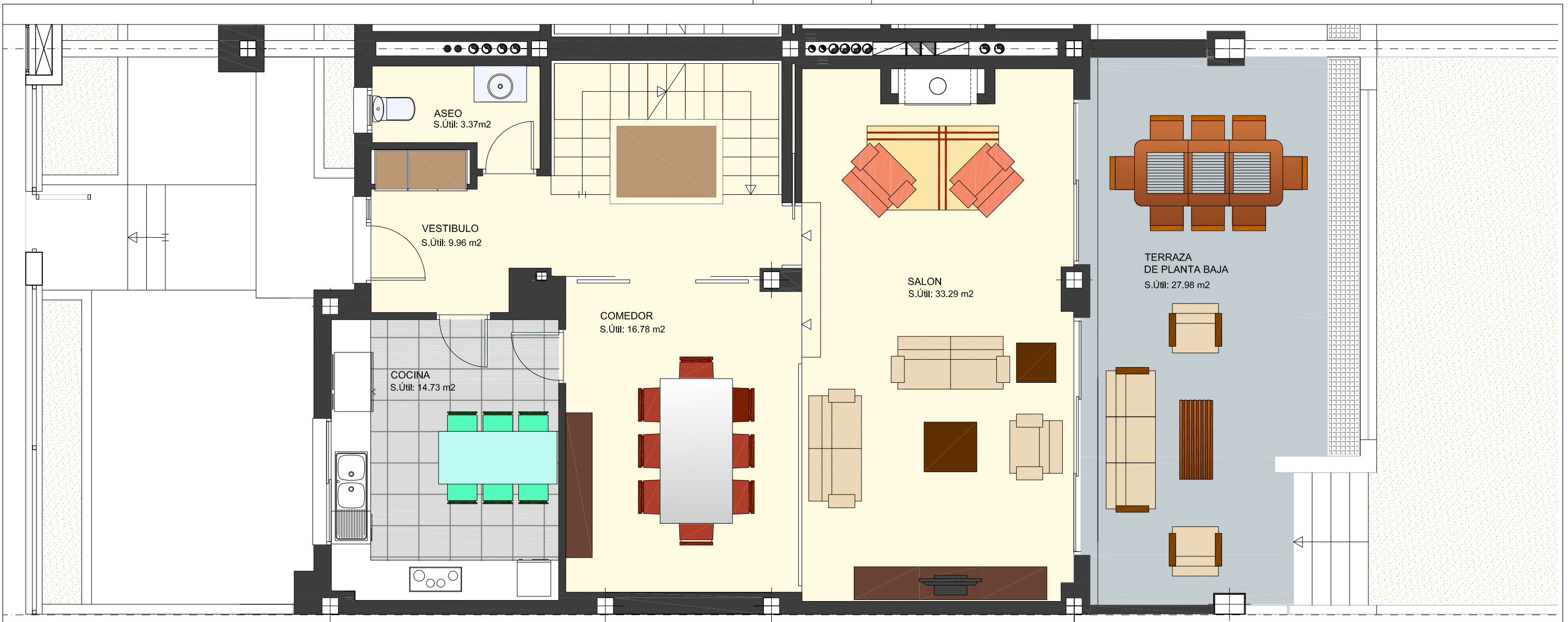
PLANTA BAJA
