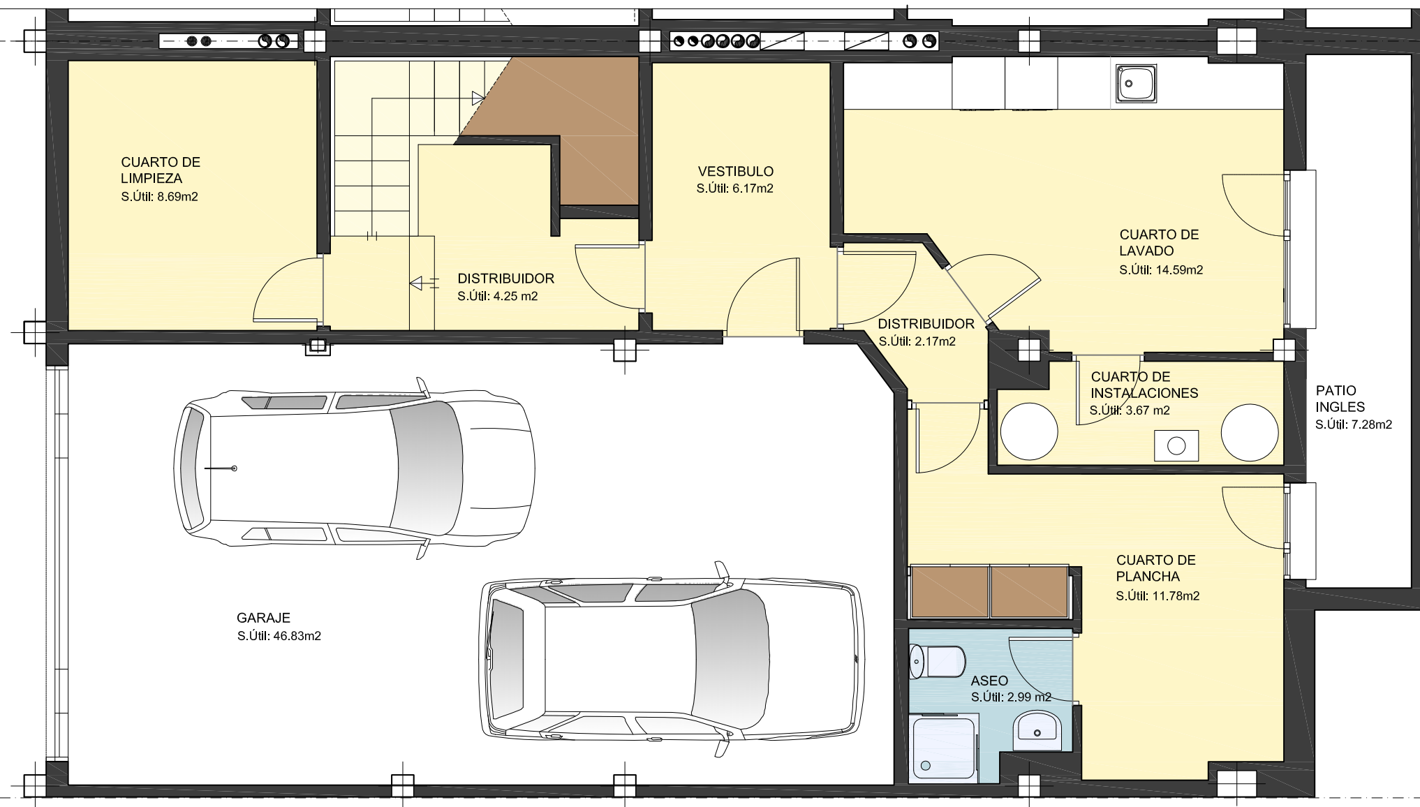
PLANTA SOTANO
