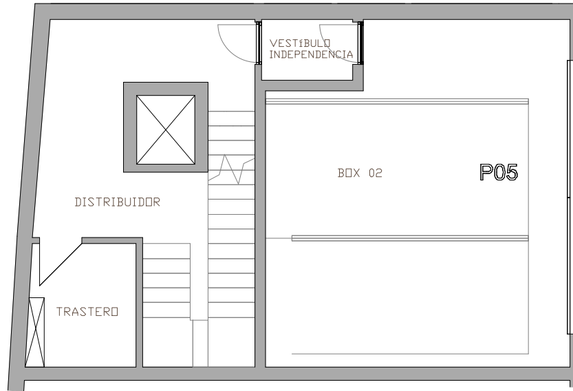
PLANTA SÓTANO
