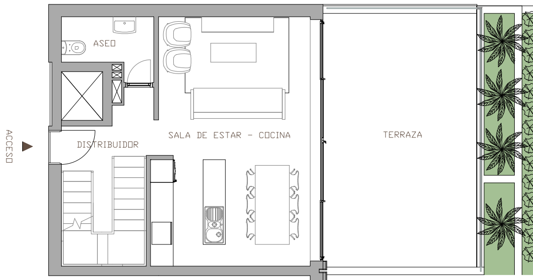
PLANTA BAJA
