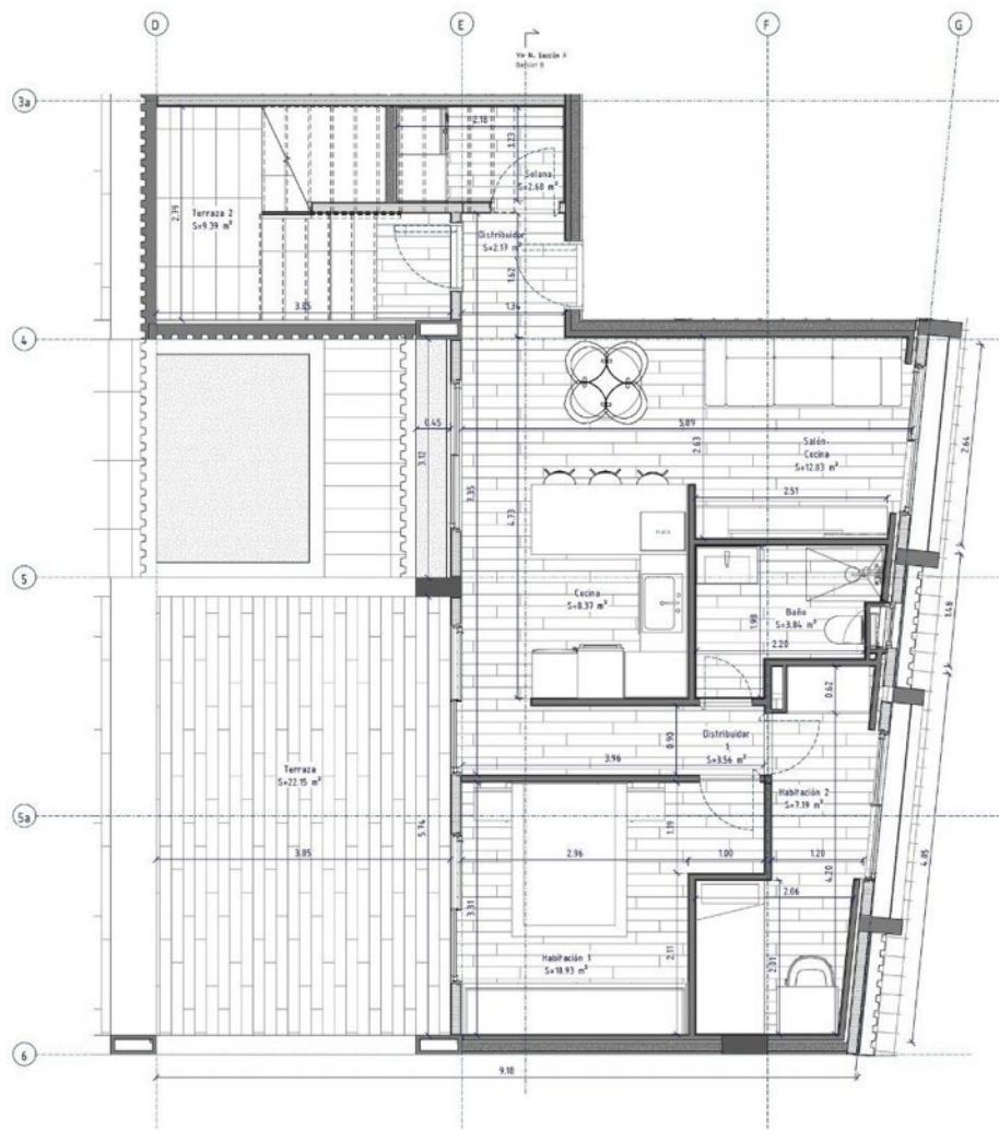
1 Vivienda 14, Planta Dossier 1:30
