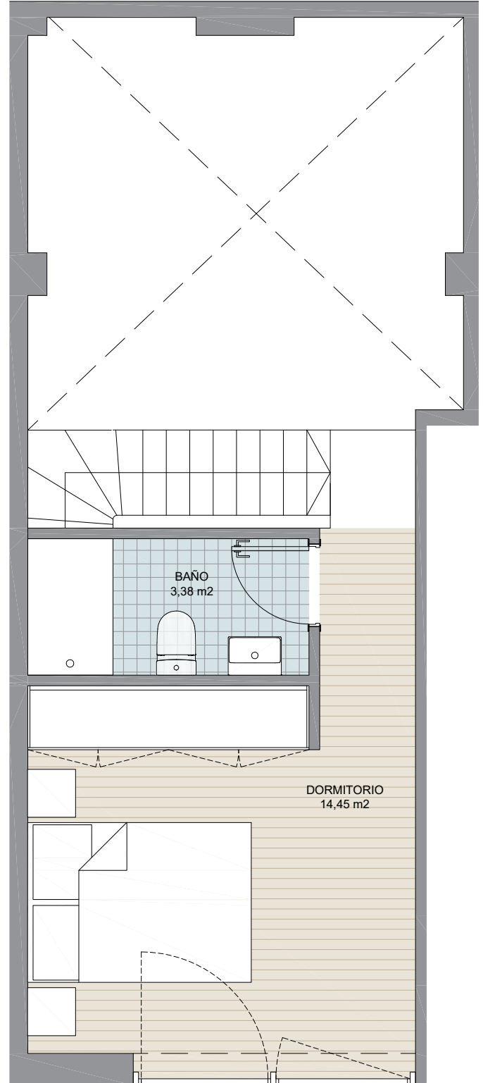
Planta alta
