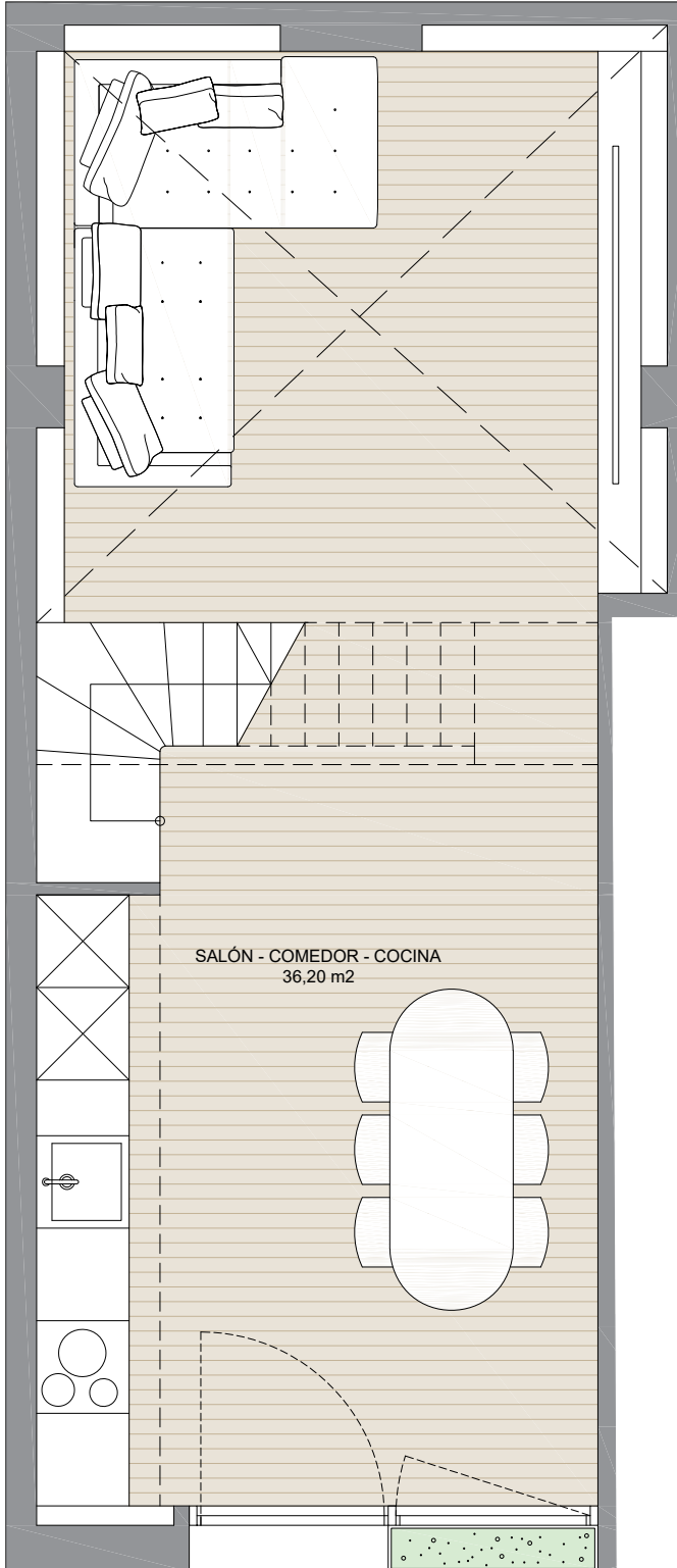
Planta baja
