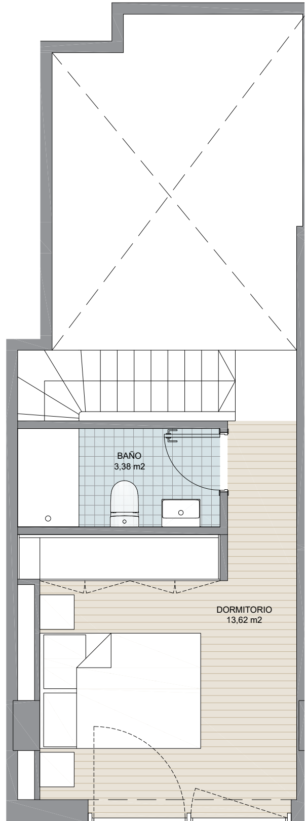
Planta alta
