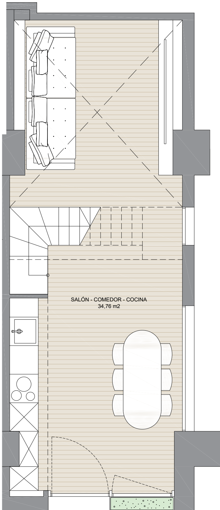
Planta baja
