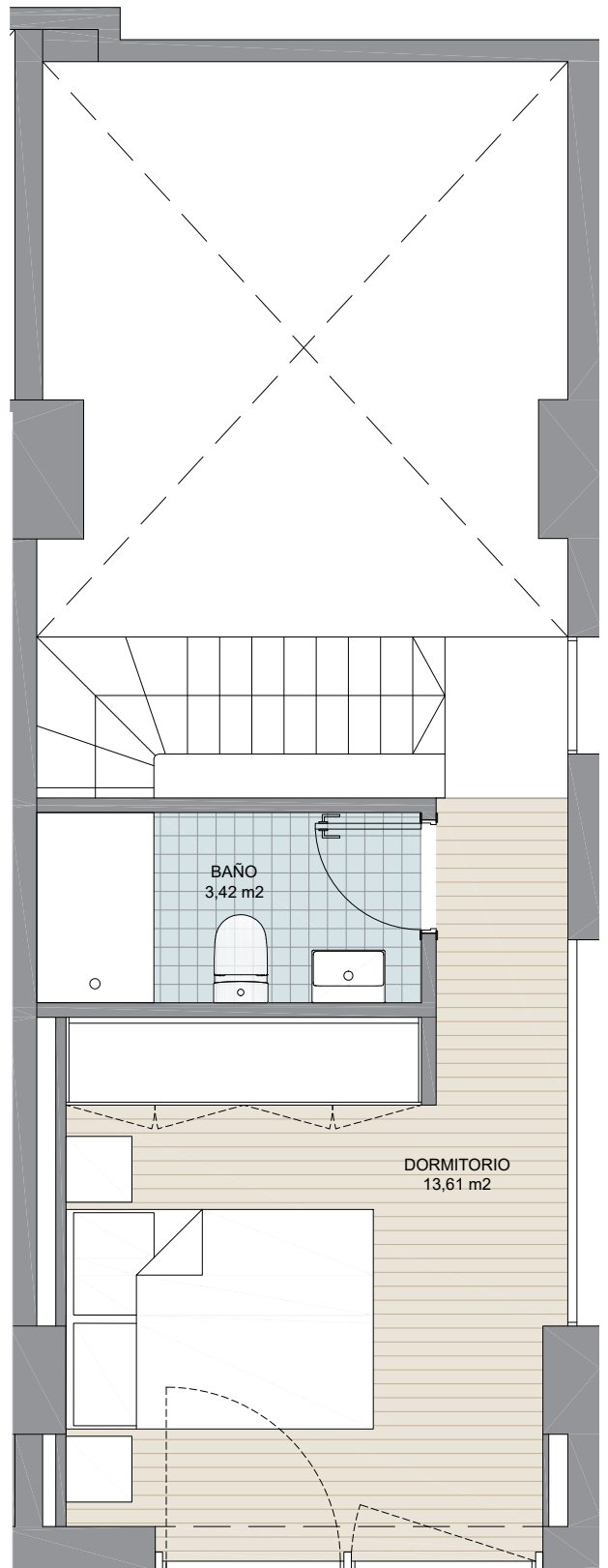
Planta alta
