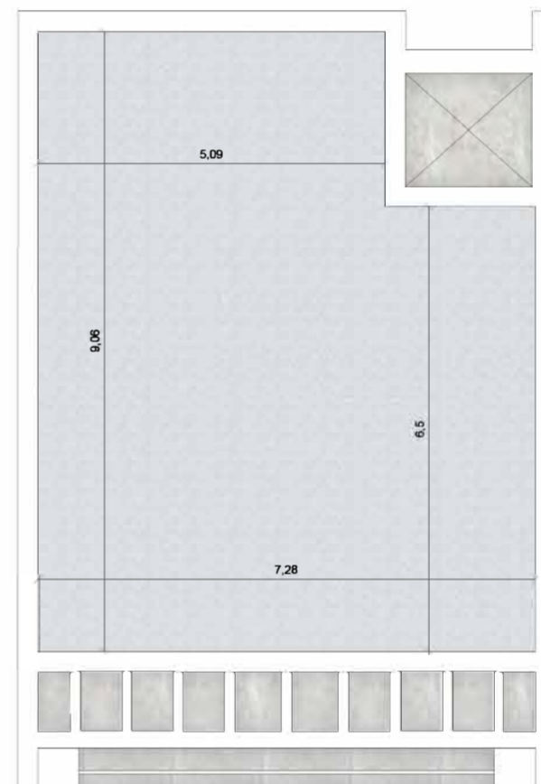
PLANTA DE CUBIERTA
